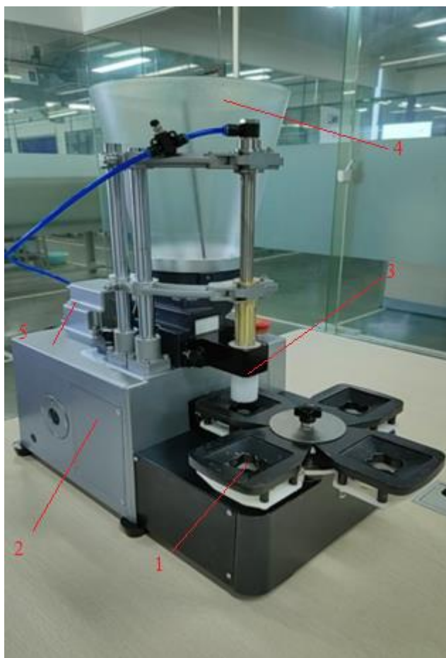
Рис1 Основные элементы управления
